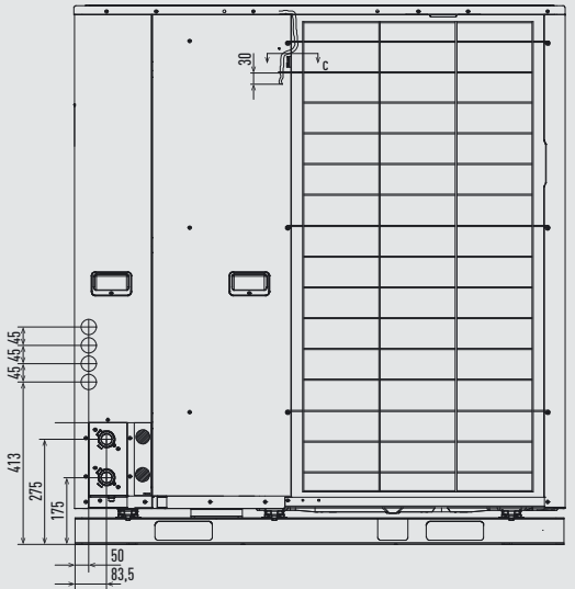
Widok z tyłu
