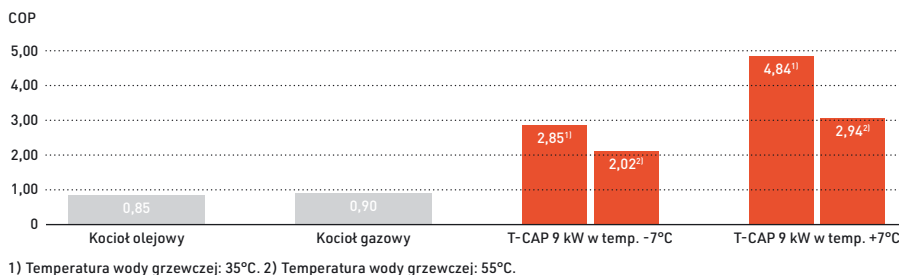
1) Temperatura wody grzewczej: 35°C. 2) Temperatura wody grzewczej: 55°C.
